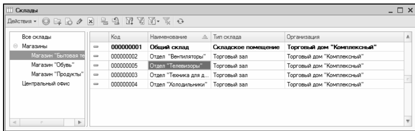
Рис. 2.16. Справочник складов
