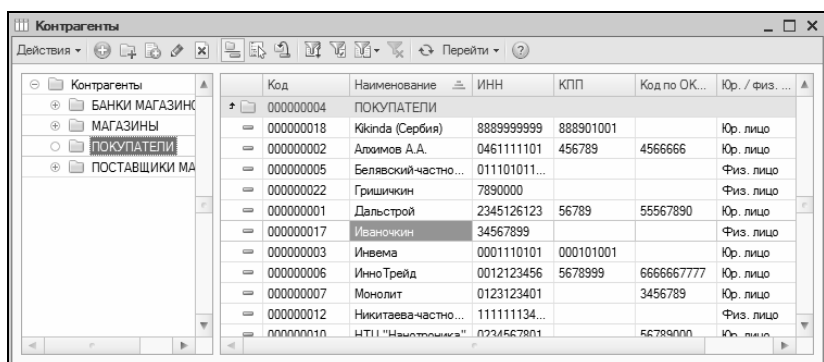
Рис. 2.11. Справочник контрагентов
