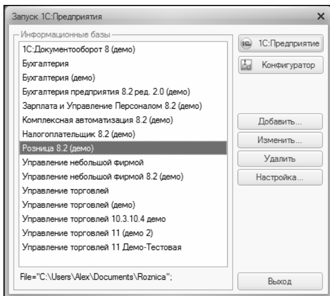
Рис. 1.1. Запуск программы
