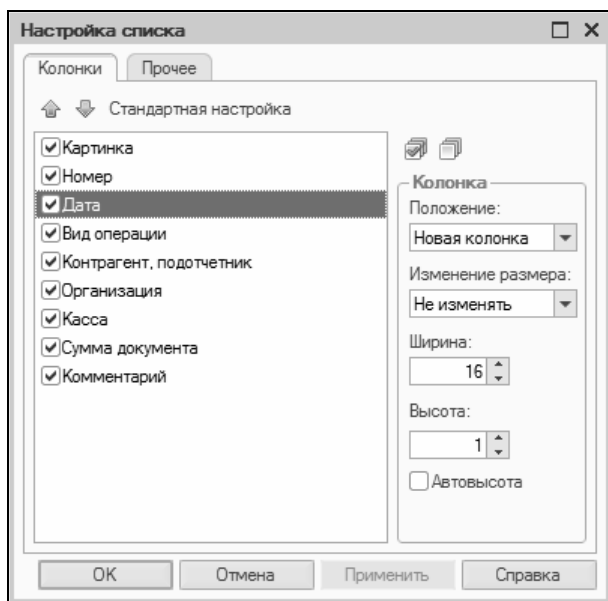
Рис. 1.18. Настройка списка
