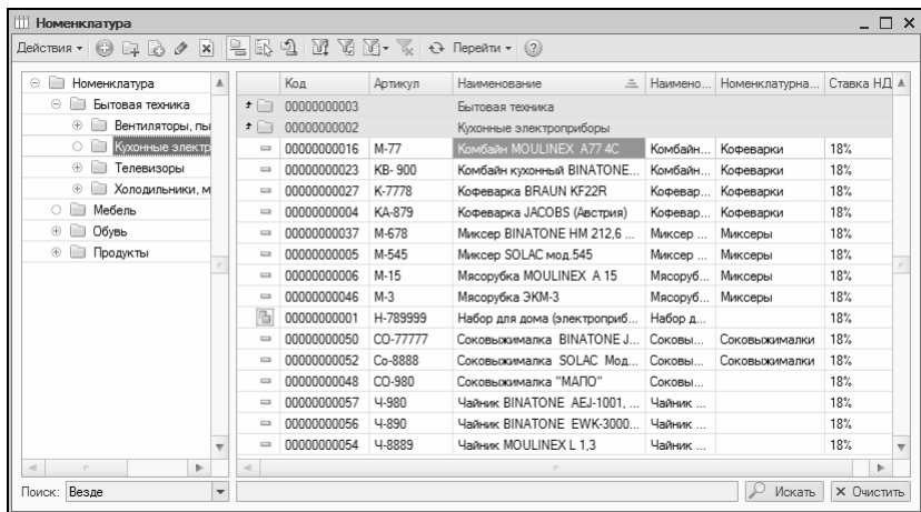
Рис. 2.23. Справочник номенклатуры
